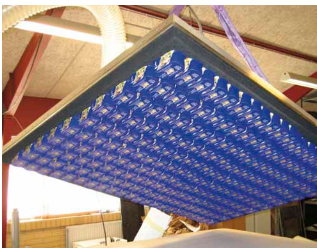
VUSS vakuum specialløft af konservesdåser.
