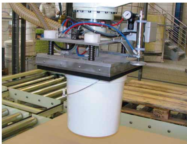
Spanden med maling løftes sikkert af VUSS vakuum systemet.
