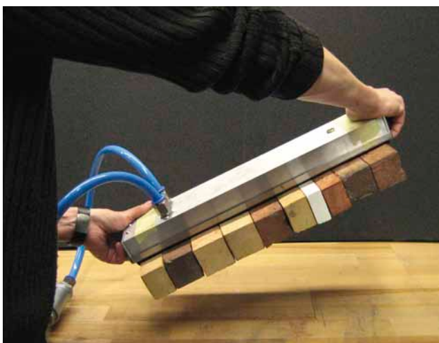
VUSS vakuum systemet kan uden omprogrammering løfte emner med forskellig overflade.
